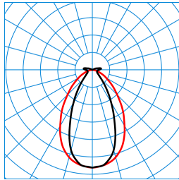
AragFHE 15 PN 100-865 ETDD PC TX782604
