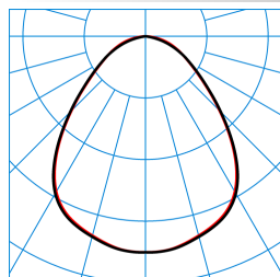
7651IP MironaF B 130-840ET L150 01ESG (LEO1) TX306204
