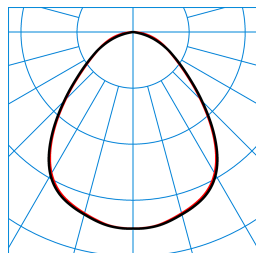
7651IP MironaF B 130-840ET L150 01ESG (LEO2) TX306231
