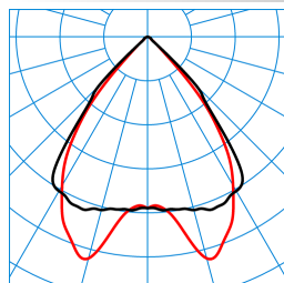
SFlow D2-L MRX LED4000-840 ET 03 TX723892
