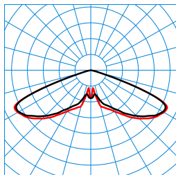
Publisca P1-RB6L-LRA/3200-740 4G1S ET (CLO initial value) TX300980
