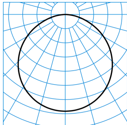
Skeo Circ MultiLC WD1 1G1Y ET +HFS E3 (nw) ■ C0 - C180 TX773615
