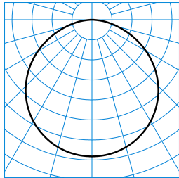
Skeo Circ MultiLC WD1 1G1Y ET +HFS E3 (ww) ■ C0 - C180 TX773680
