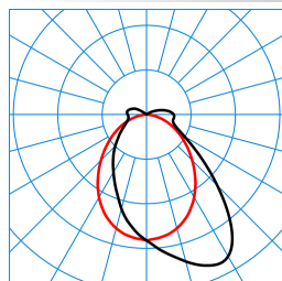
AragF 6 PAW 20-840 ET PC EB3 TX774513
