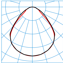
ValineoG4 M73 PW19 38-50/4ML-830 ET X2 (stage 0) TX773238
