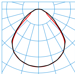
ValineoG4 M73 PW19 38-50/4ML-830 ET X2 (stage 2) TX773266
