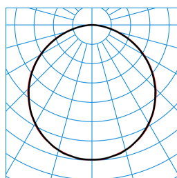
Olisq QWD3 DW 30-840 ETBLE +DMM IP54 IK + Olisq QWD3 ZDR 1/1 03 TX460938
