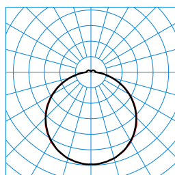
Olisq QWD3 DW 30-840 ETBLE +DMM IP54 IK + Olisq QWD3 ZDR 1/2 05 TX462017
