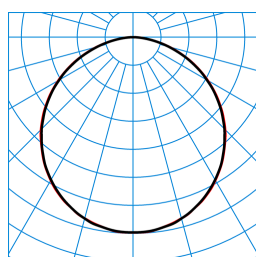
Olisq QWD3 DW 30-840 ETBLE +DMM IP54 IK + Olisq QWD3 ZDR 1/1 01 TX461618
