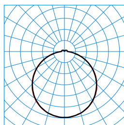
Olisq QWD3 DW 30-840 ETBLE +DMM IP54 IK + Olisq QWD3 ZDR 1/2 03 TX460711
