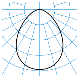
InperlaL G2 C07 HR22 2700-830 01 + DA-M 01 ■ C0 - C180 TX053075
