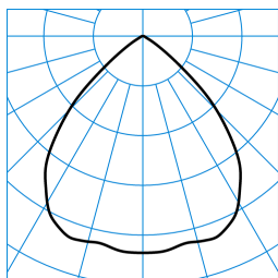
InperlaL G2 C07 HR22 2700-830 01 + RD-PC ■ C0 - C180 TX053076
