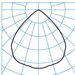
InperlaL G2 C07 HR22 2700-830 01 + DA 01 ■ C0 - C180 TX053074
