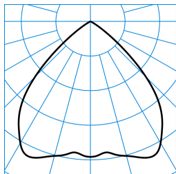
InperlaL G2 C07 HR22 2700-830 ETDD 01 ■ C0 - C180 TX769933
