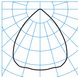
InperlaL G2 C07 HR22 2700-830 01 + ZN-PC ■ C0 - C180 TX053078
