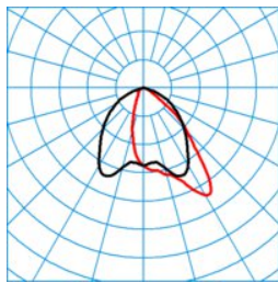
Jovie 70-AM3L-24-240-740-CLO-B
