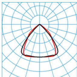
ELINE LW2240-110 ML 830 L150 2 20 ■ C0 - C180
