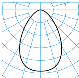
InperlaL G2 C07 HR19 1800-840 03 + DA-M 03 ■ C0 - C180 TX053021
