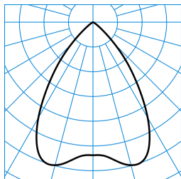
InperlaL G2 C07 HR19 1800-840 03 + DA 03 ■ C0 - C180 TX053020
