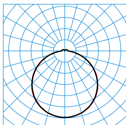
Olisq QWD3 DW 30-840 ET EB3 IP54 + Olisq QWD3 ZDR 1/2 05 TX461155
