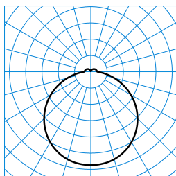
Olisq RWD1 DW 10-840 ET IP54 + Olisq RWD1 ZDR 1/2 03 TX428600
