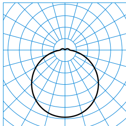
Olisq RWD1 DW 10-840 ET IP54 + Olisq RWD1 C 01 TX425604
