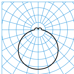
Olisq RWD1 DW 10-840 ET IP54 TX375500
