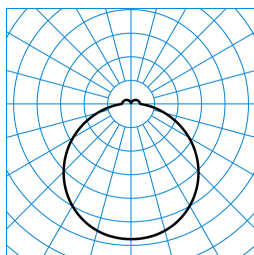
Olisq RWD1 DW 10-840 ET IP54 + Olisq RWD1 ZDR 1/2 01 TX425668
