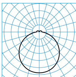
Olisq RWD1 DW 10-840 ET IP54 + Olisq RWD1 ZDR 1/2 05 TX428752
