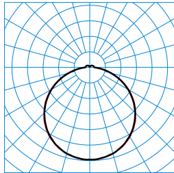
Olisq QWD2 DW 20-840 ETBLE +DMM IP54 + Olisq QWD2 ZDR 1/2 01 TX461172
