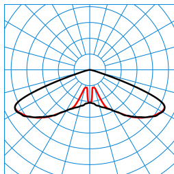
Publisca P2-RB6L-LR/1000-730 2G1S ET (CLO initial value) TX301684
