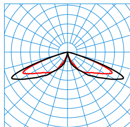
LTX K-RB6L-LR/1200-730 2G1 ET TX780475
