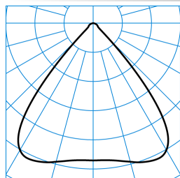
Mirona Fit R LW 150-840 ET TX843249
