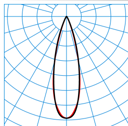
7650 L-SHB 230V CEAG L37 01 TX768848
