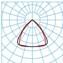
ELINE LW2255-140 ML 830 L225 4 20 ■ C0 - C180
