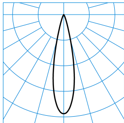
7651 Lentyp L-SP 40-835 M34 ETBLE 05 (225) TX782551
