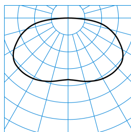
PolaroniQ WD1-2 LED3000-830 + WD2 C1 TX773835
