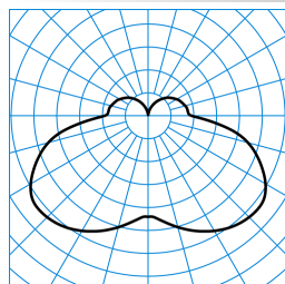
PolaroniQ WD1-2 LED3000-830 ET TX773837
