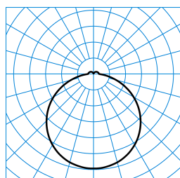
Olisq RWD3 DW 30-840 ET EB3 + Olisq RWD3 ZDR 1/2 05 TX426416
