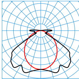
Nextrema G3 B 6000-840 ETDD PC TX770365
