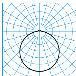
Olisq RWD2 DW 14-40/4/ML-830 ET + Olisq RWD2 ZDR 1/2 01 (stage 0) TX776630
