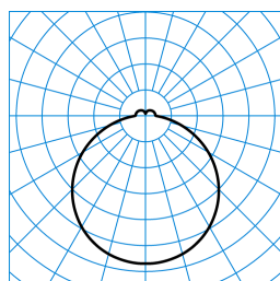
Olisq RWD2 DW 14-40/4/ML-830 ET (stage 3) TX776613
