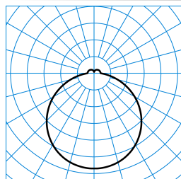
Olisq RWD2 DW 14-40/4/ML-830 ET (stage 0) TX776610
