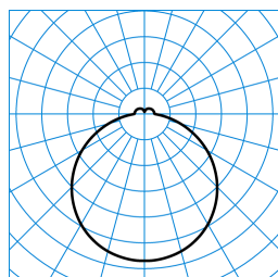
Olisq RWD2 DW 14-40/4/ML-830 ET (stage 1) TX776611
