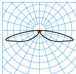
LTX PT-SB3L-LR/1500-740 2G1 ET TX776795
