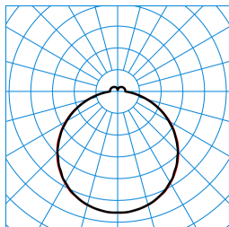
Olisq QWD2 DW 35-840 ETBLE +DMR IP54 IK TX777542
