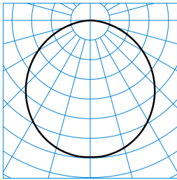
Olisq RWD2 DW 20-830 ET HFS IP54 PC + Olisq RWD2 ZDR 1/1 01 TX425890
