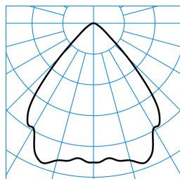
InperlaLP C05 HR25 2700-840 03 + DA 01 TX041788
