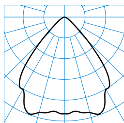
InperlaLP C05 HR25 2700-840 03 + RD-PC TX041792
