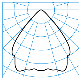
InperlaLP C05 HR25 2700-840 03 + RG-PC TX041793
