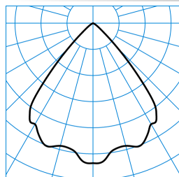
InperlaLP C05 HR25 2700-840 ET 03 TX771431
