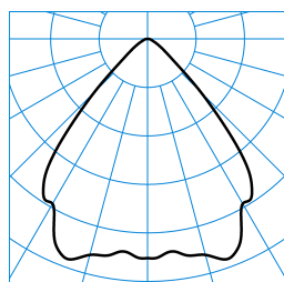
InperlaLP C05 HR25 2700-840 03 + DA 03 TX041789
