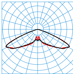
Publisca P1W-RB6L-LR/3800-740 6G1S ET (CLO end value) TX301215
