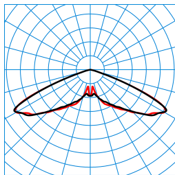
Publisca P1W-RB6L-LR/3800-740 6G1S ET (CLO initial value) TX300290
