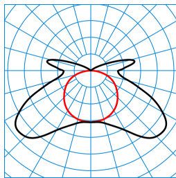
AragF 12 PXW 20-64/16ML-840 ET PC (stage 10) TX770010
