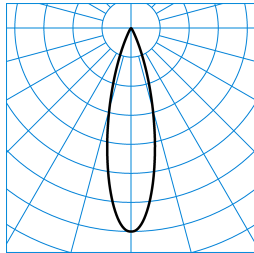
7651 LentyP L-MF 40-EW M48 ET 03 (225) TX782199
