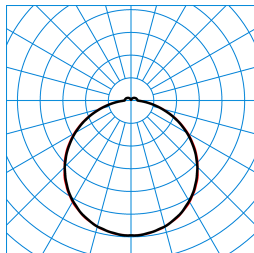
Olisq QWD3 DW 30-830 ETDD IP54 + Olisq QWD3 ZDR 1/2 01 TX461813
