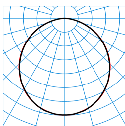
Olisq QWD3 DW 30-830 ETDD IP54 + Olisq QWD3 ZDR 1/1 01 TX461820
