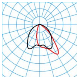
Jovie 70-AM3L-12-135-730-CLO-B
