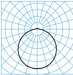
Olisq RWD2 DW 20-8TW ETBLE +CAS IP54 + RWD2 ZDR 1/2 05 (DWW) TX873489
