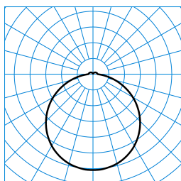
Olisq RWD2 DW 20-8TW ETBLE +CAS IP54 + RWD2 ZDR 1/2 03 (DWW) TX873486
