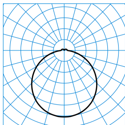
Olisq RWD2 DW 20-8TW ETBLE +CAS IP54 + RWD2 ZDR 1/2 01 (DWW) TX873483
