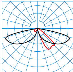
LTX P-AB2L-LRA/15/18/26-740 4G1 (1500 lm) TX059699
