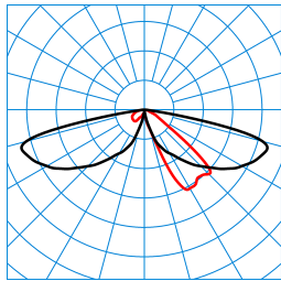
LTX P-AB2L-LRA/15/18/26-740 4G1 (1800 lm) TX062701
