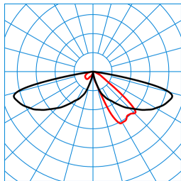
LTX P-AB2L-LRA/15/18/26-740 4G1 (2600 lm) TX062702
