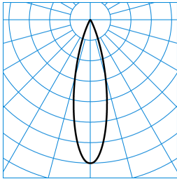
7651 Lentyp L-MF 40-EW M48 ETBLE 03 (150) TX782201
