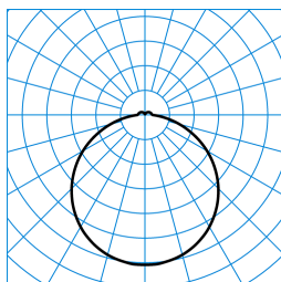
Olisq RWD2 DW 20-830 ETDD + Olisq RWD2 ZDR 1/2 03 TX427745
