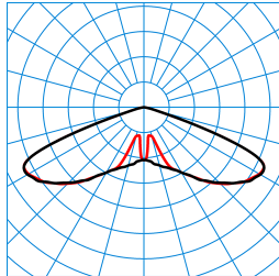
Publisca P2-RB6L-LRA/1000-740 2G1S TX047880
