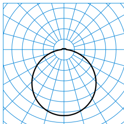
Olisq RWD4 DW 60-830 ETBLE +DMM IP54 PC + Olisq RWD4 ZDR 1/2 01 TX427314
