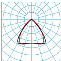
ELINE LN40-110 ML 830 L150 4 20
