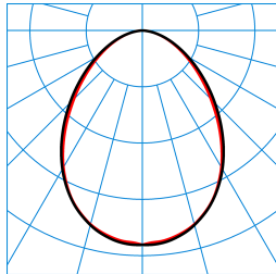
SFlow D1-L MRWD LED3200-830 ETDD 03 TX769750
