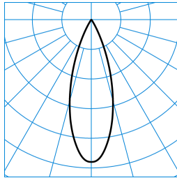
7651 LentyP L-FL 40-827 M32 ETDD 05 (150) TX781802
