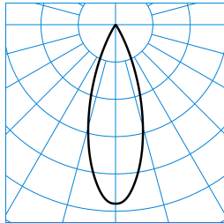
7651 LentyP L-FL 40-827 M32 ETDD 05 (225) TX781803
