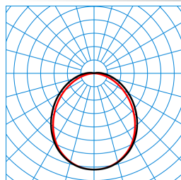
3331 G2 D2 TS LED3700-840 ET 01 TX771009
