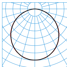
Olisq QWD3 DW 45-830 ET IP54 IK + Olisq QWD3 ZDR 1/1 03 TX461363
