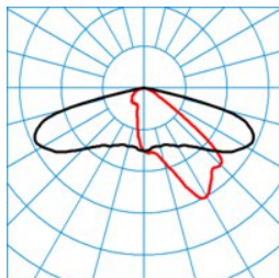
Jovie 50-AB2L-6-68-740-CLO-B
