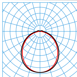
4401 G2 C15 DW IP 40-830 ET TX773621
