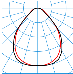
ArmoFit G2 M52 PW 20-830 ETBLE +CAS TX558480
