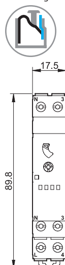
Type 14.61 Push-in aansluiting
