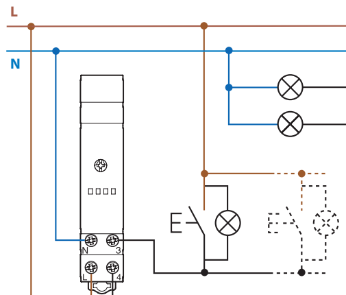
4-draads aansluiting (L verbonden met drukknop)
