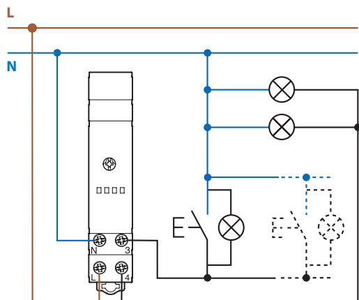
3-draads aansluiting (N verbonden met drukknop)*
