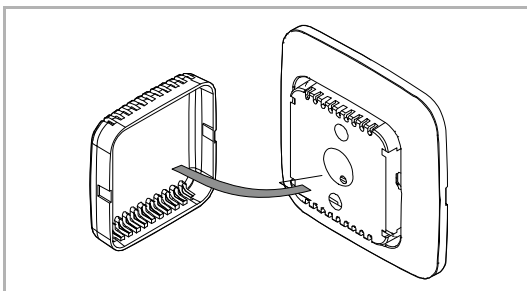
Fig. 13: Montar la cubierta
