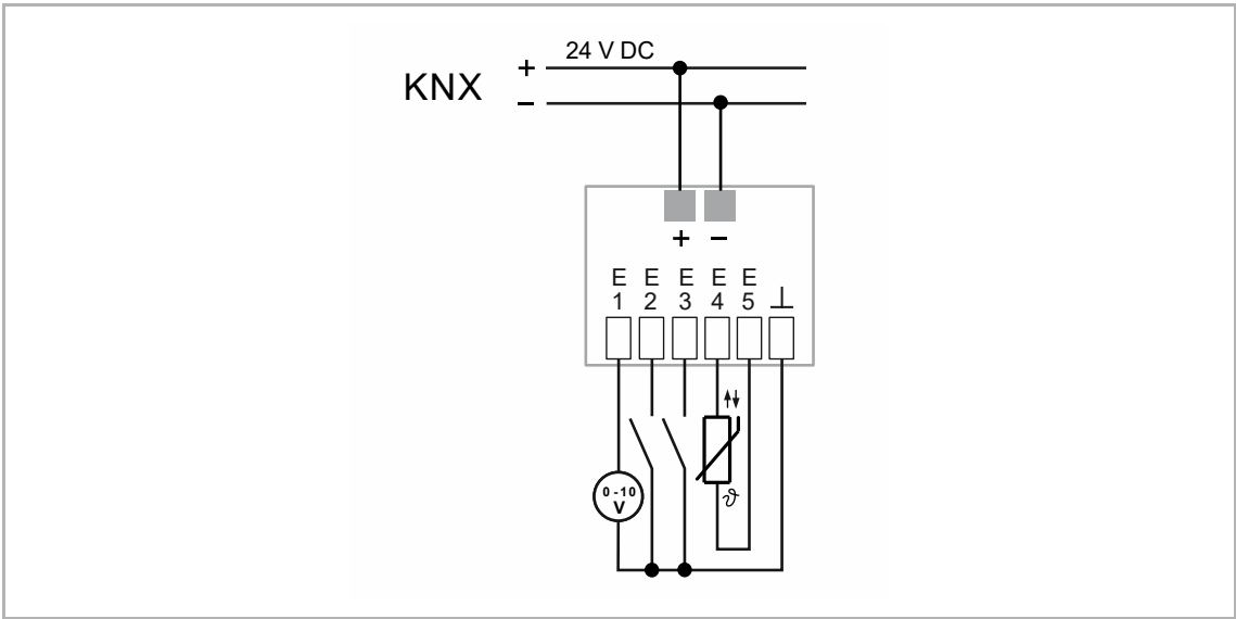
Fig. 14: Conexión eléctrica
