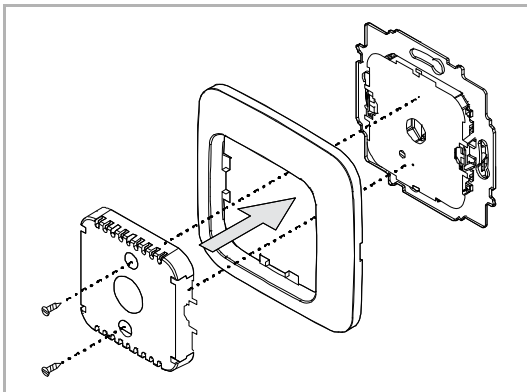
Fig. 12: Montaje del elemento superior
