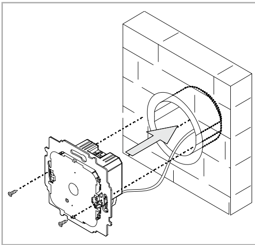
Fig. 11: Montar el elemento empotrable
