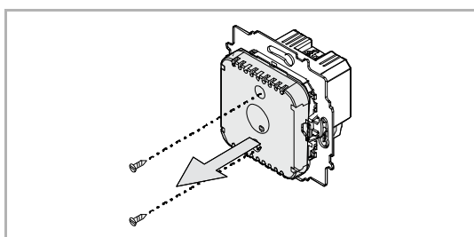
Fig. 9: Estado de entrega: extraer el elemento de control
